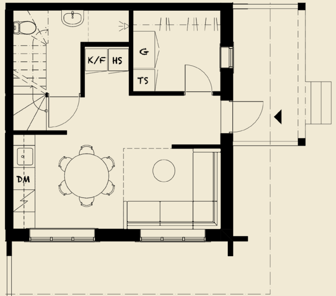
ENTRÉPLAN
