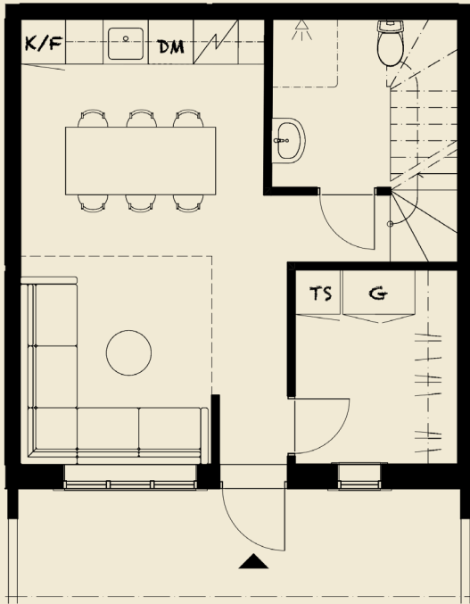
ENTRÉPLAN
